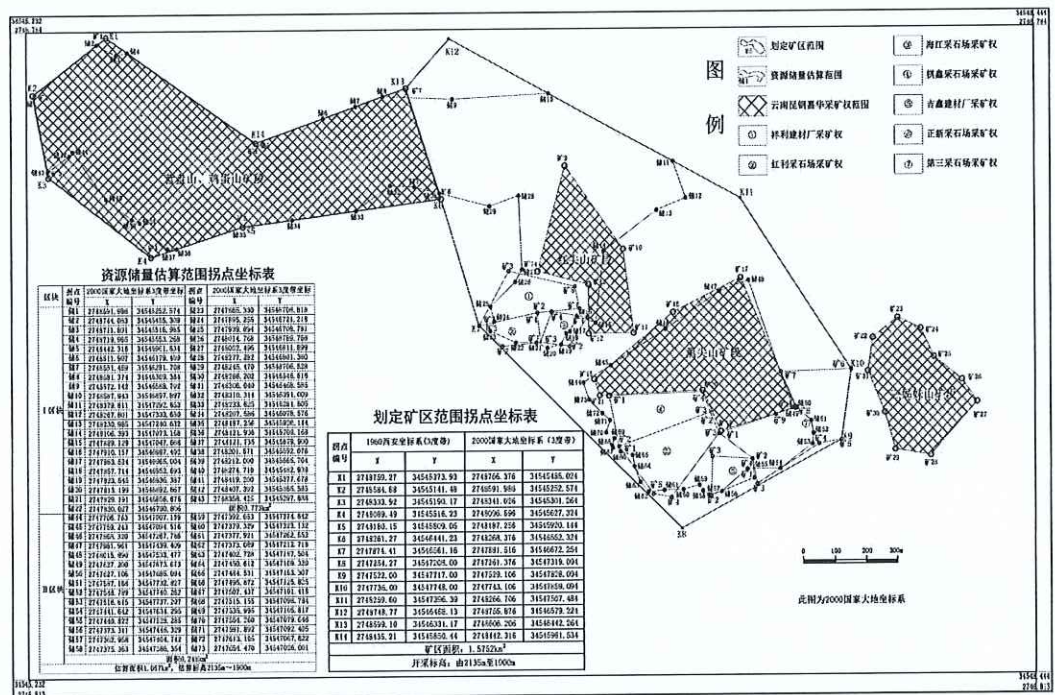
图1 矿界示意图
