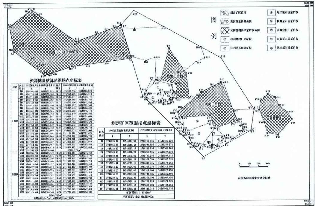
图1 矿界示意图
