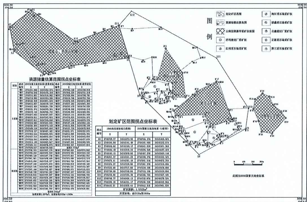
图1 矿界示意图
