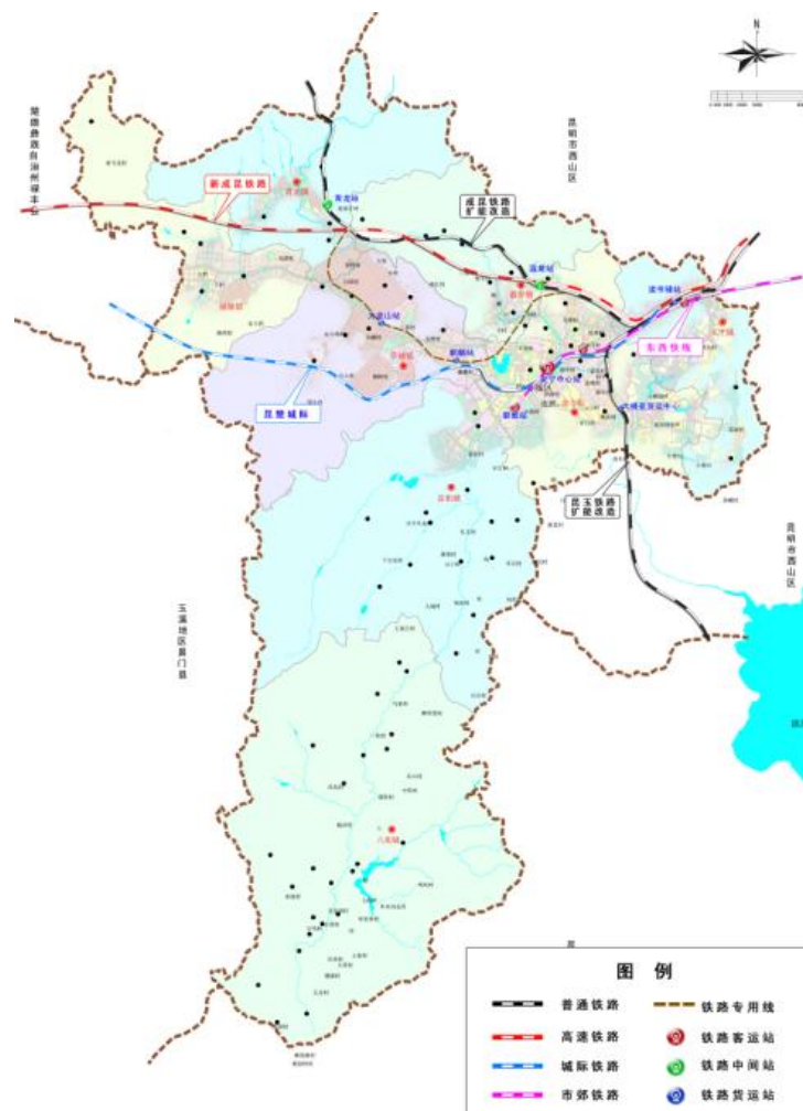
图 4-13 安宁市规划铁路线路走向
