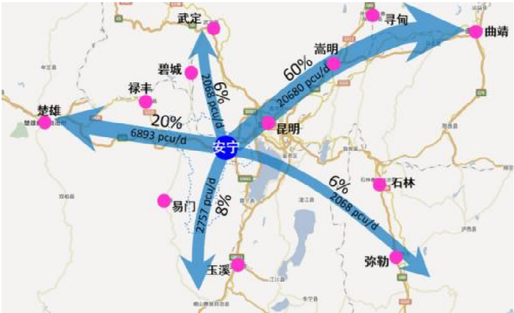
图 2-6 2020 年市域对外交通分布图（不含过境）
