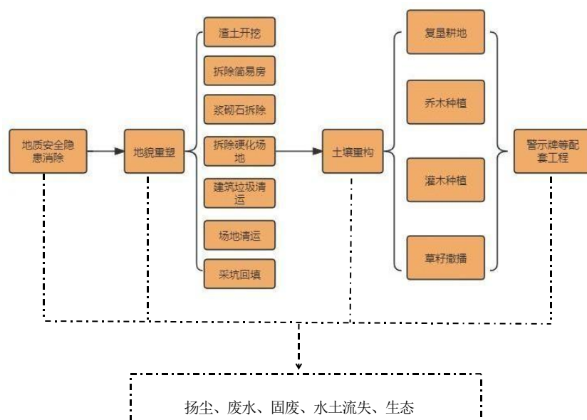
图 4-1 项目施工工艺流程及污染环节图
