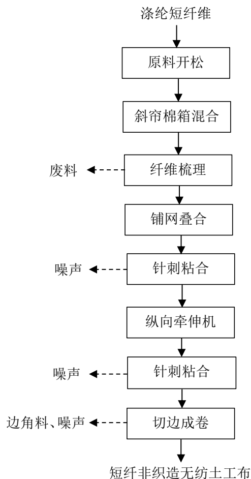
图 2-12 短纤非织造无纺土工布生产工艺及产污环节图
