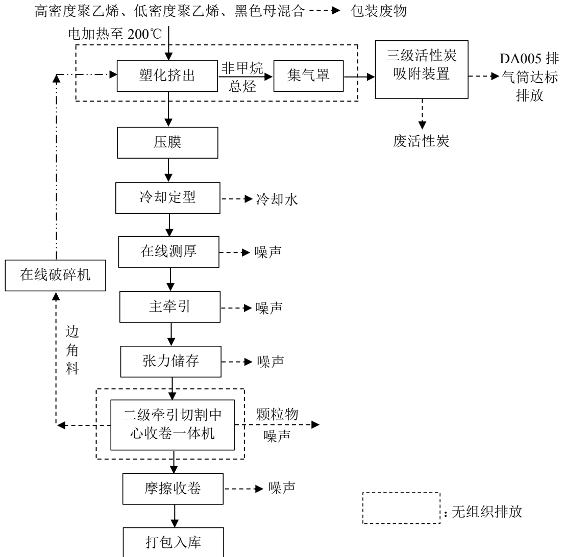
图 2-6 压延土工膜生产工艺流程及产污环节图
