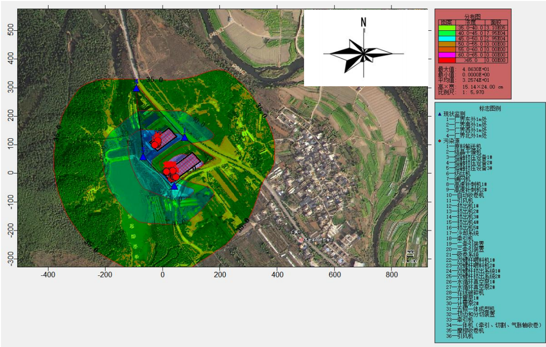
图 4-2 项目运营期噪声贡献值等级线分布图
