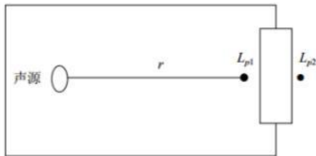
图 4-1 室内声源等效为室外声源示意图
