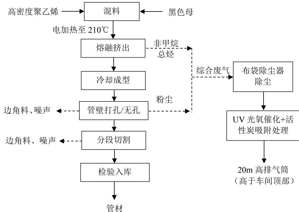
图 2-18 管材生产工艺及产污环节图
