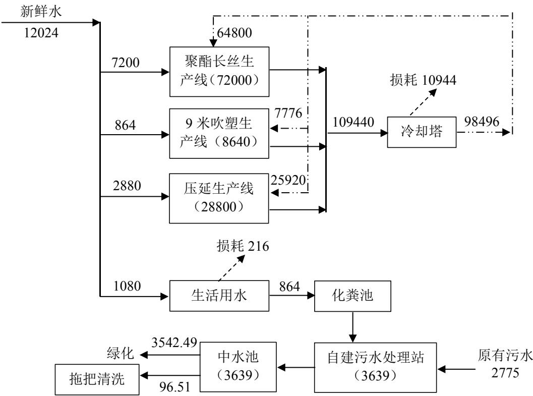
图 2-1 产能扩建项目晴天水量平衡图 单位：m³/a
