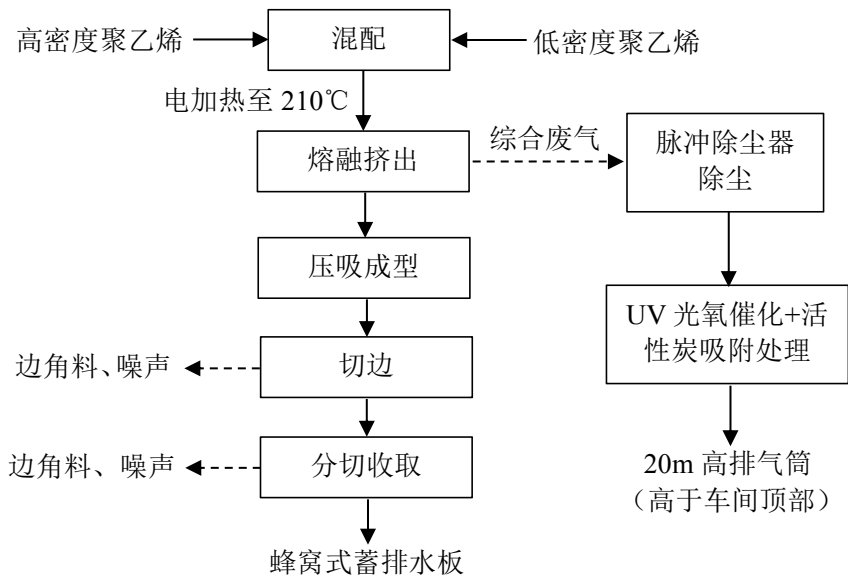
图 2-15 蜂窝式蓄排水板生产工艺及产污环节图
