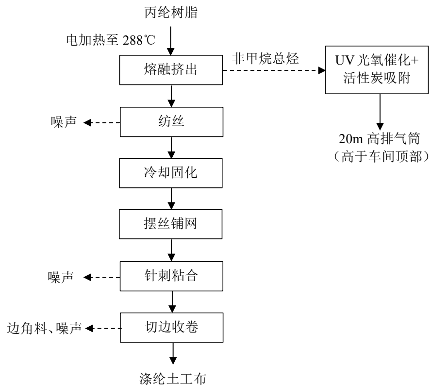
图 2-10 涤纶土工布生产工艺及产污环节图
