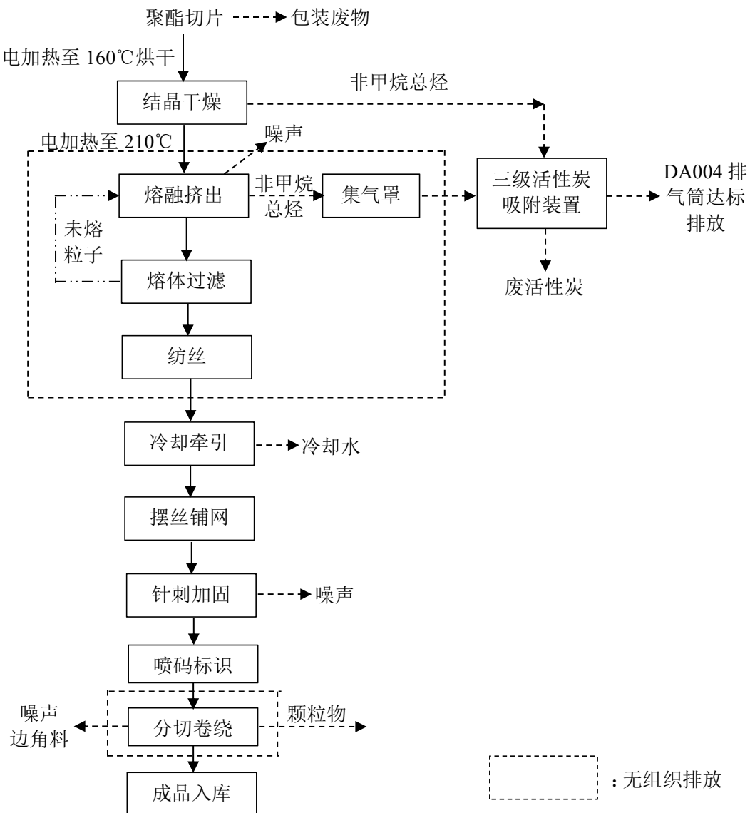
图 2-4 聚酯长丝无纺土工布生产流程及产污环节图
