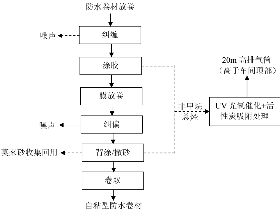
图 2-14 自粘型防水卷材生产工艺及产污环节图
