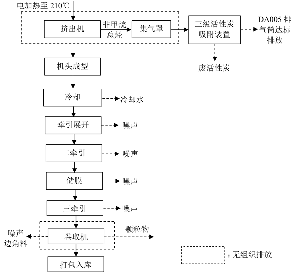
图 2-5 9 米吹塑氮糙土工膜生产工艺流程及产污环节图 工艺流程简述:
