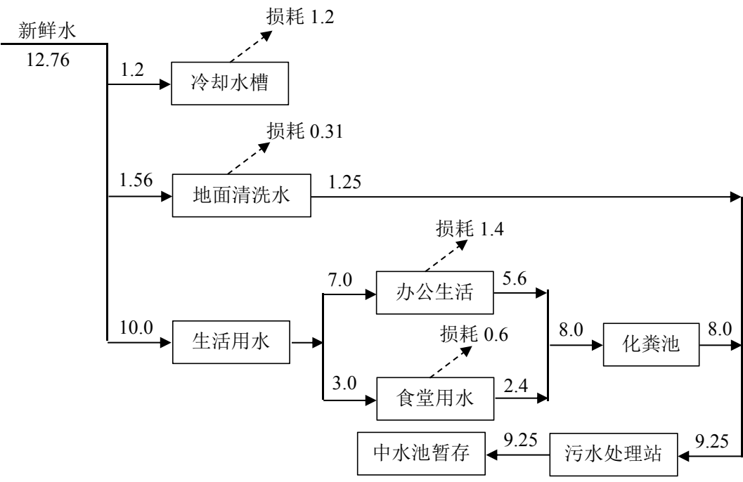
图 2-7 原有项目雨天水量平衡图 单位：m³/d
