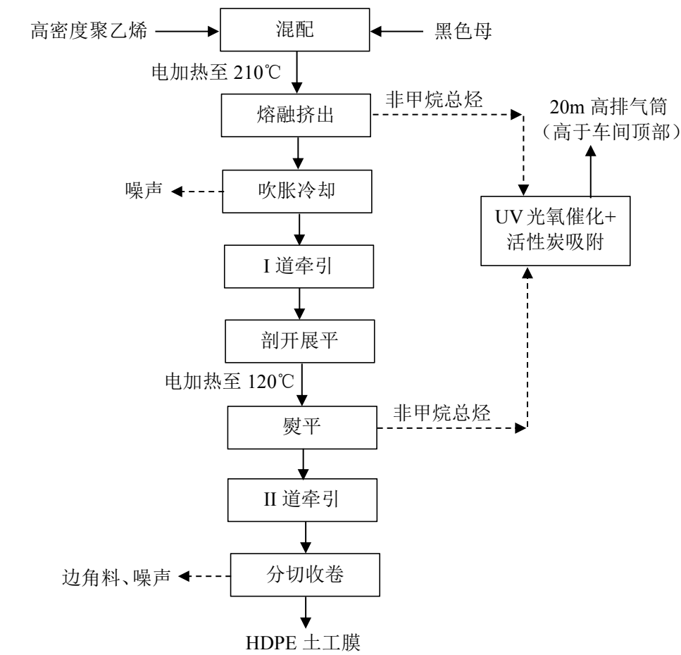
图 2-11 HDPE 土工膜生产工艺及产污环节图
