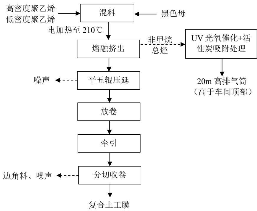
图 2-16 复合土工膜生产工艺及产污环节图
