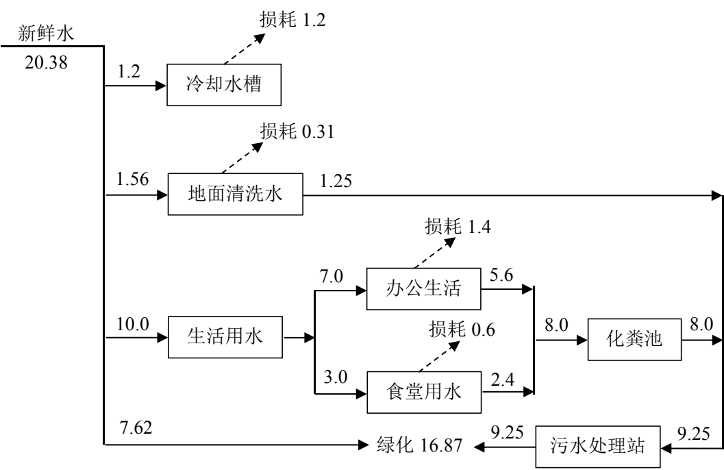
图 2-6 原有项目非雨天水量平衡图 单位：m³/d
