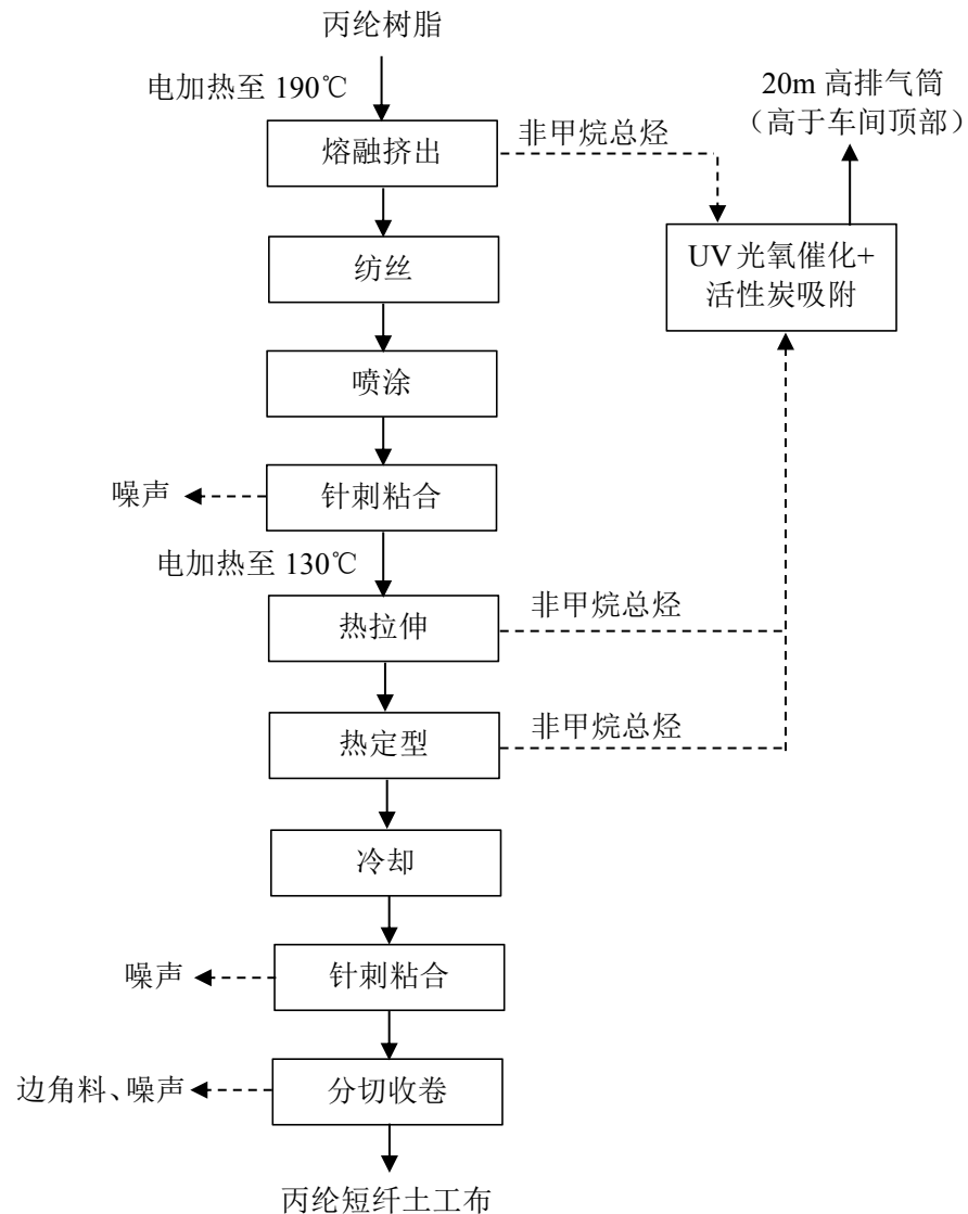
图 2-9 丙纶短纤土工布生产工艺及产污环节图
