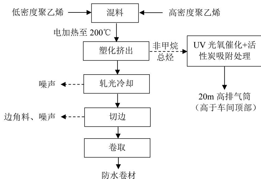
图 2-13 防水卷材生产工艺及产污环节图
