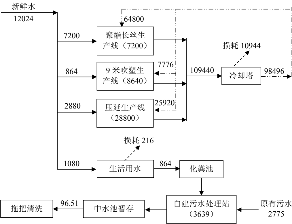
图 2-2 产能扩建项目雨天水量平衡图 单位：m³/a
