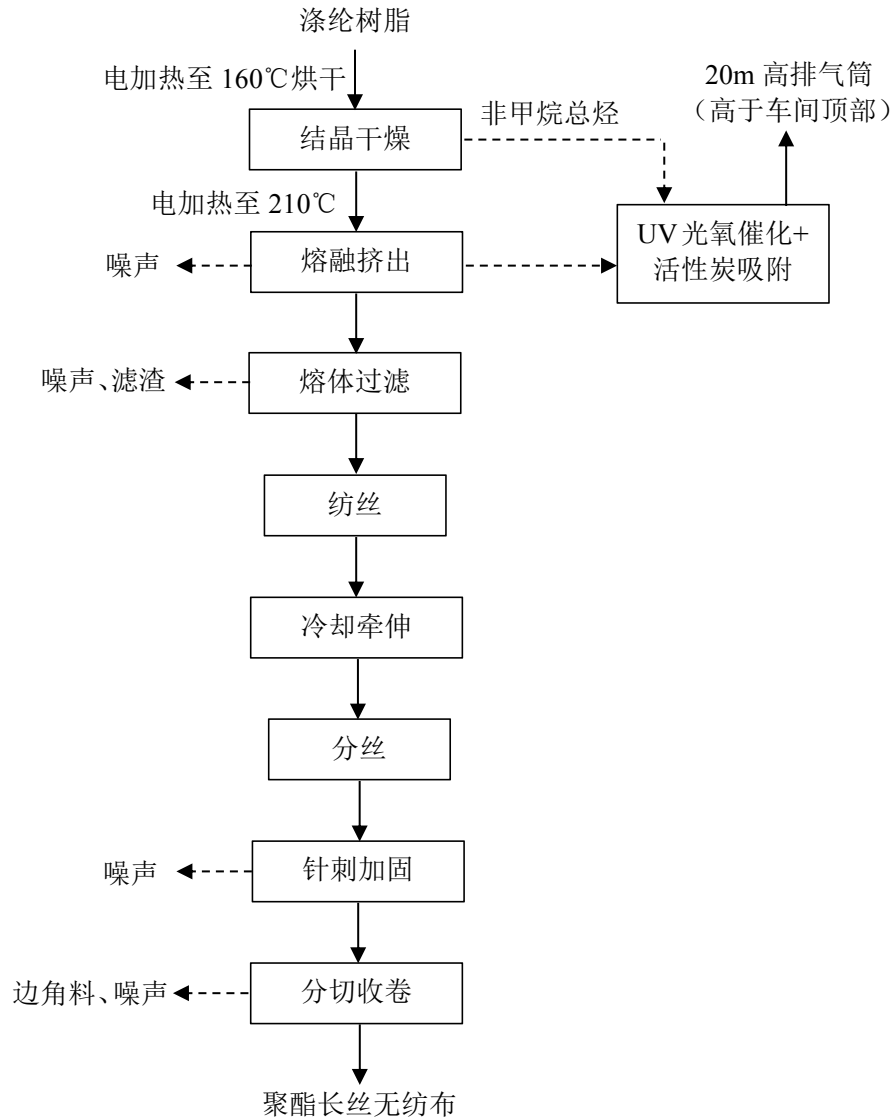
图 2-8 聚酯长丝无纺布生产工艺及产污环节图
