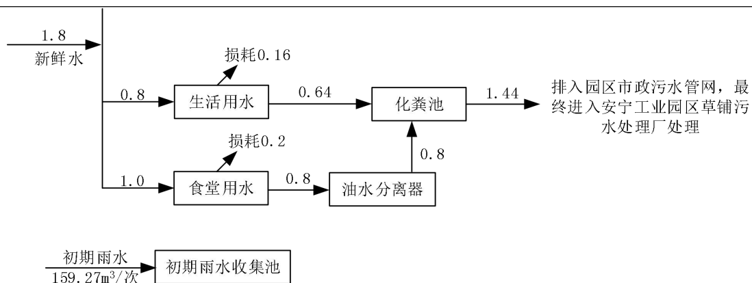
图 2-2 项目雨季水平衡图（单位：m³/d）
