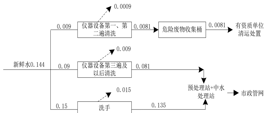
图 2-1 项目水平衡图 单位: m^3/d
