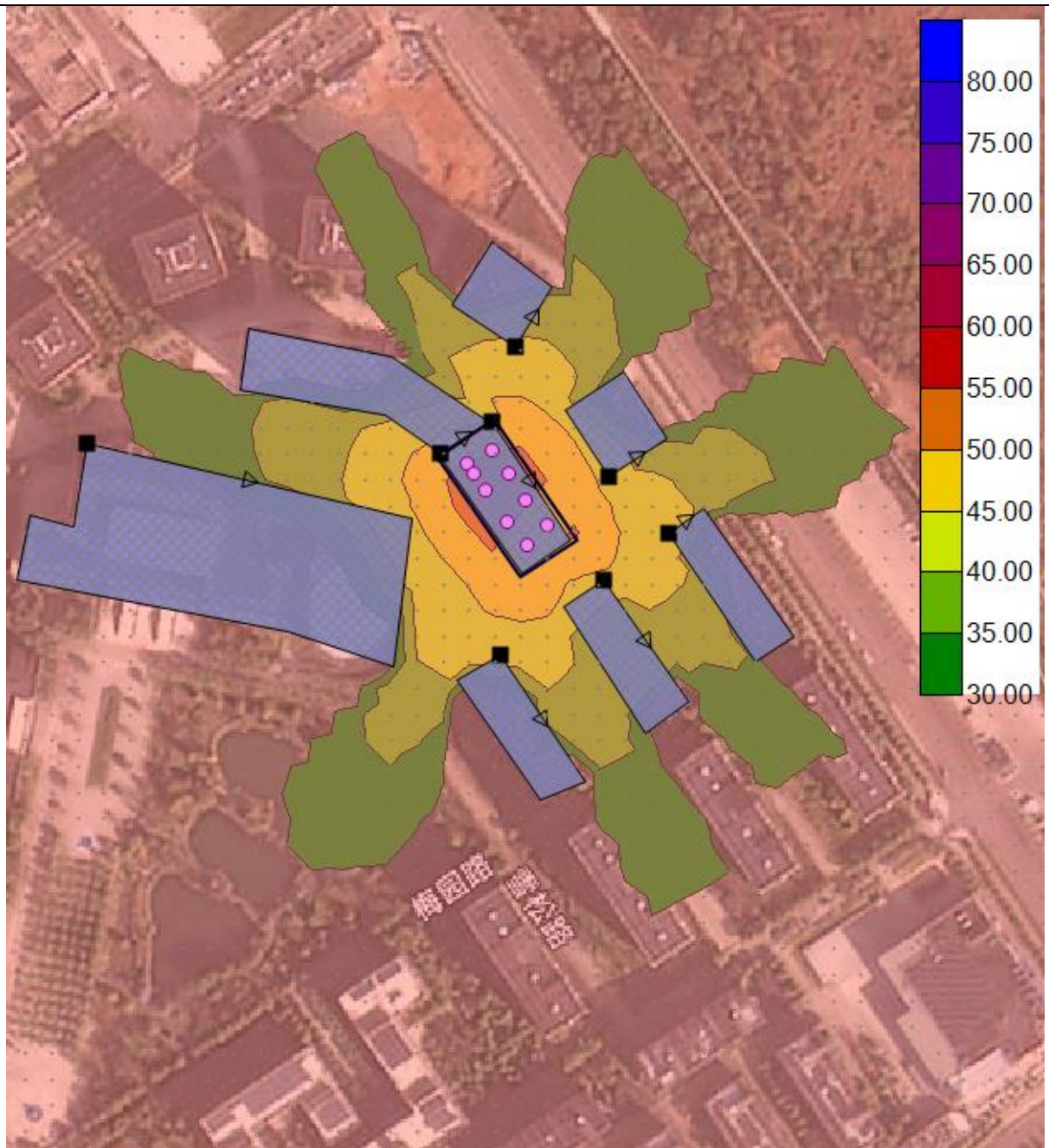
项目噪声预测等声级线图
