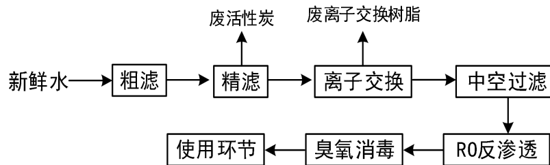
图 2-8 纯水工艺流程图
