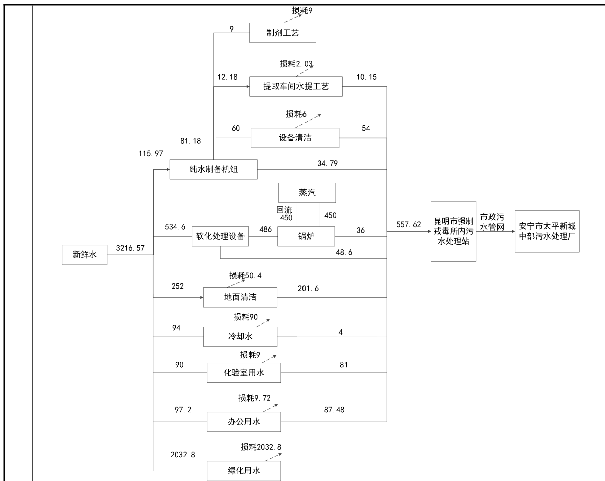
图 2-1 项目水量平衡图 (m³/a)
