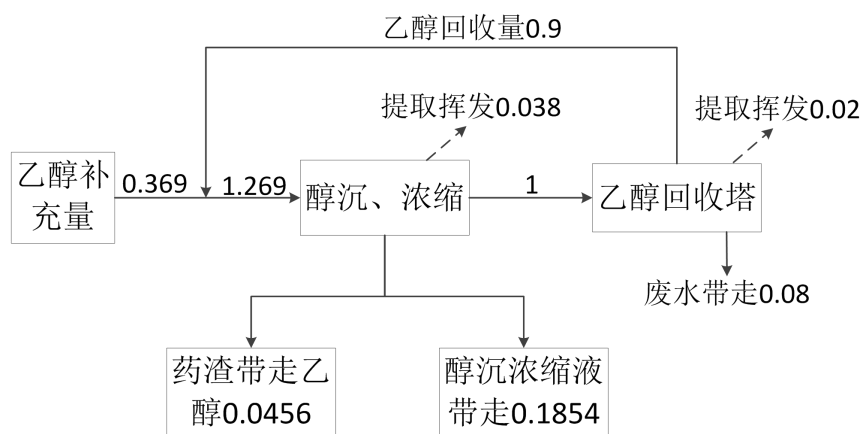
图4-1 项目乙醇平衡图（单位：t/a）
