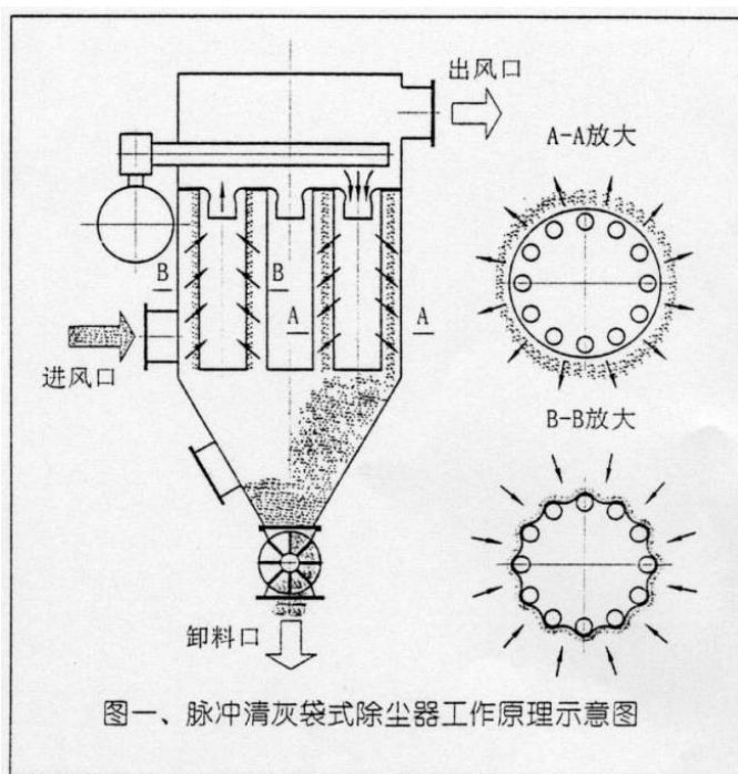
图4-2 脉冲布袋除尘器工作原理
