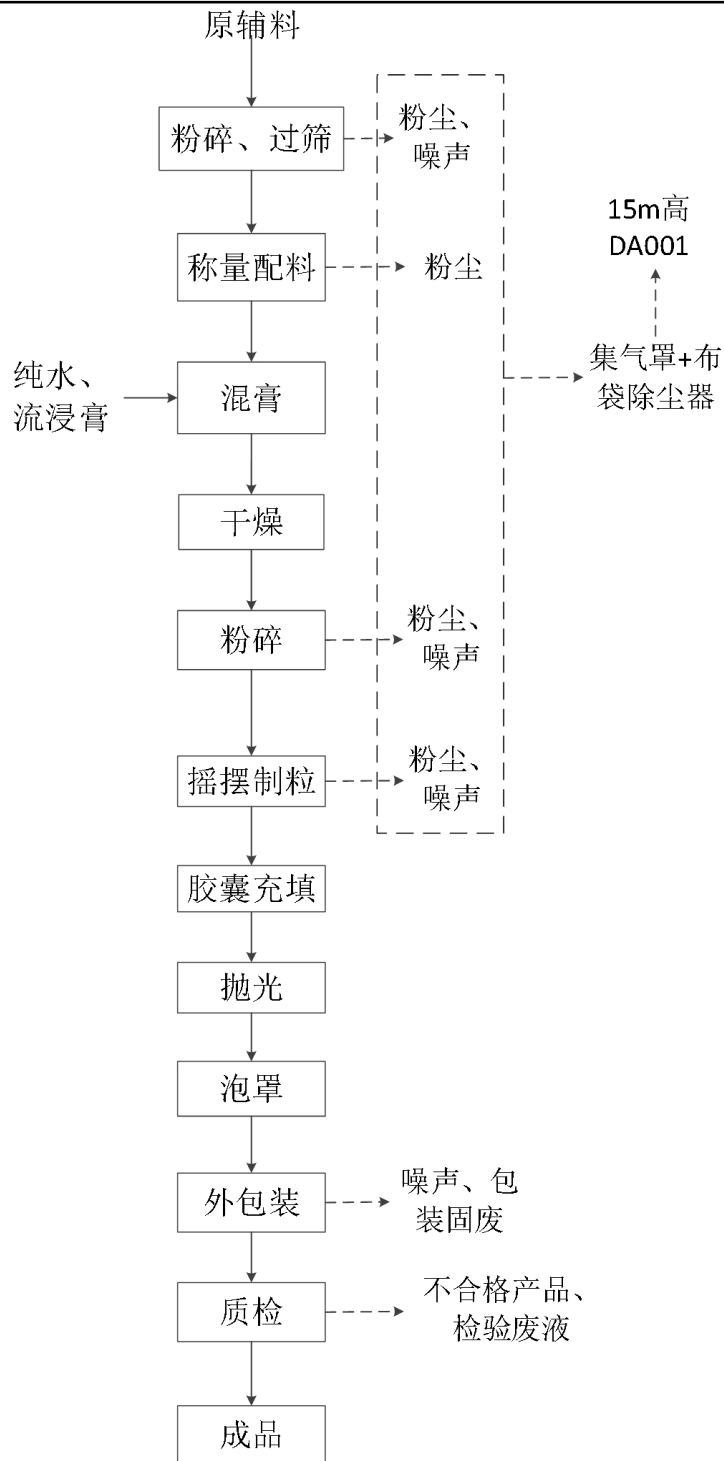
图 2-9 项目胶囊剂生产工艺流程及产排污节点图
