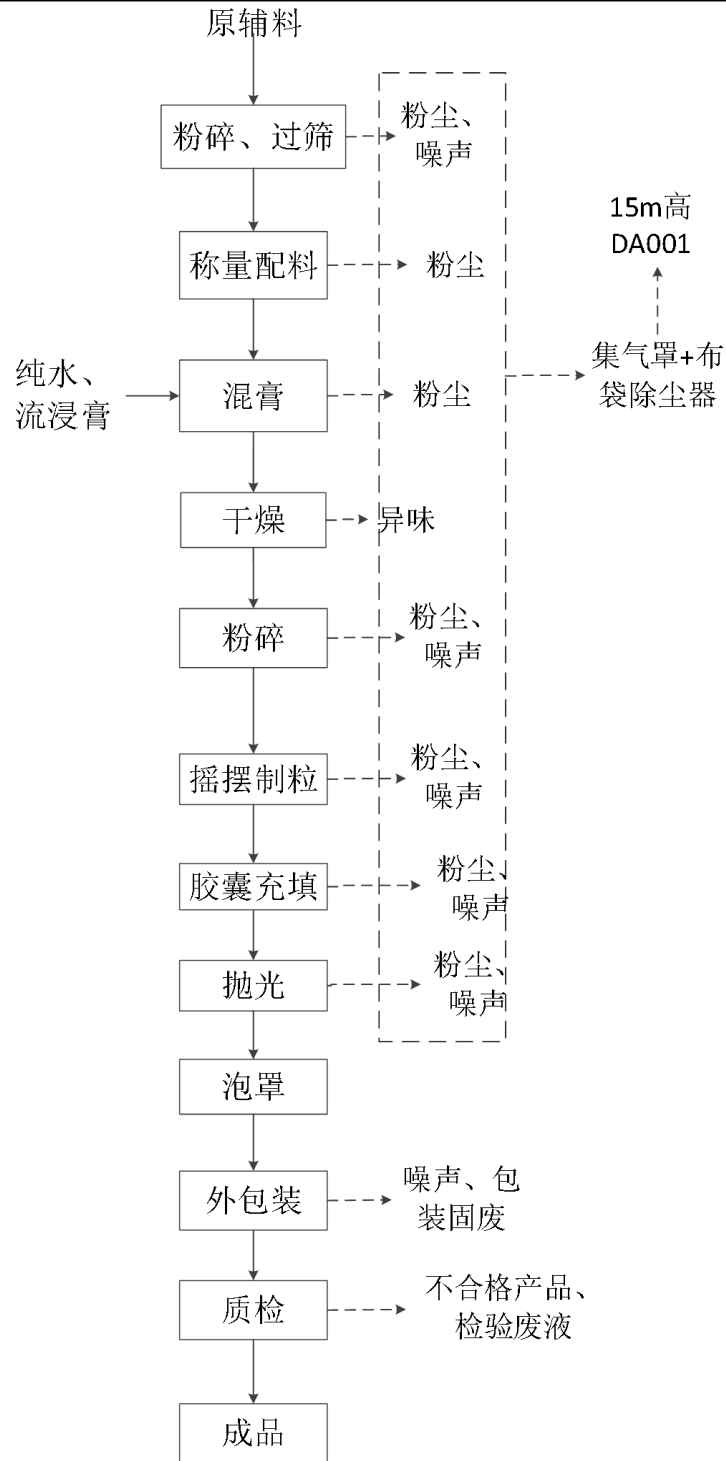
图 2-6 项目胶囊剂生产工艺流程及产排污节点图
