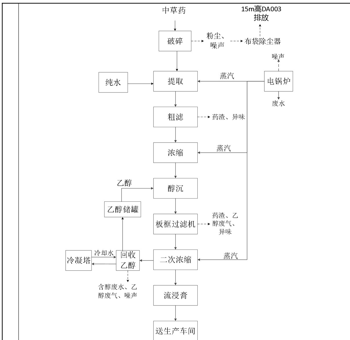
图 2-5 项目提取工序工艺流程及产排污节点图
