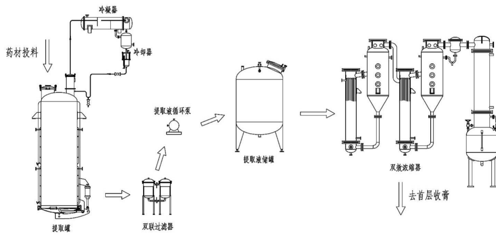
图 2-3 中药材水提浓缩（提取罐）工艺设备流程环节图
