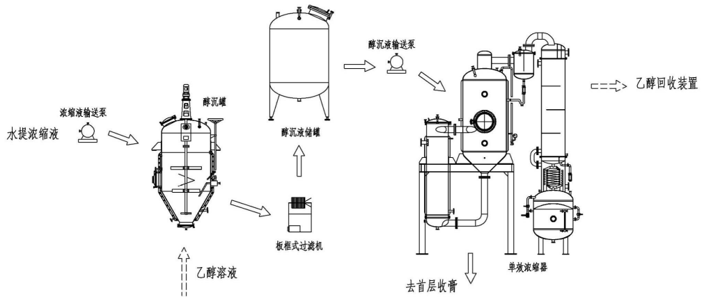
图 2-4 醇沉浓缩设备流程环节图
