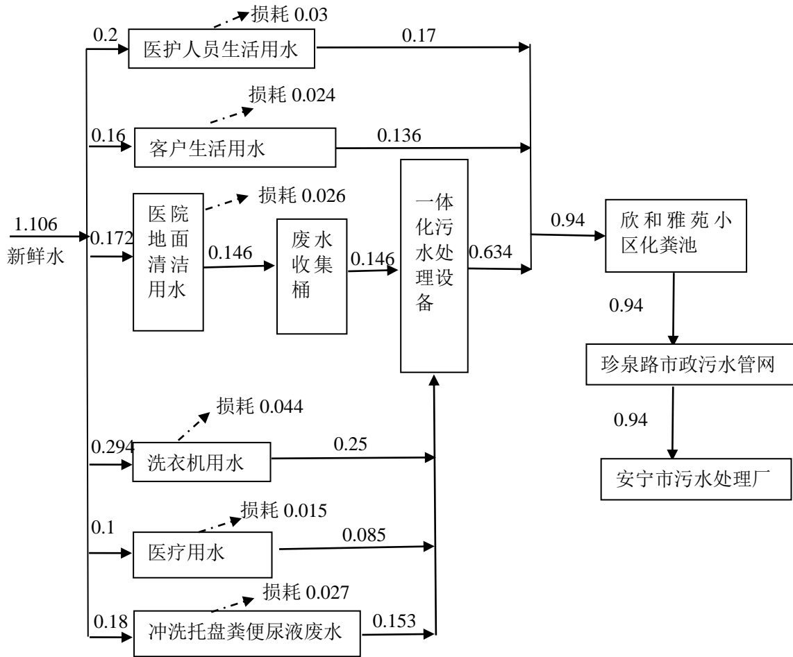
图 4-1 项目水平衡图 单位: m³/d
