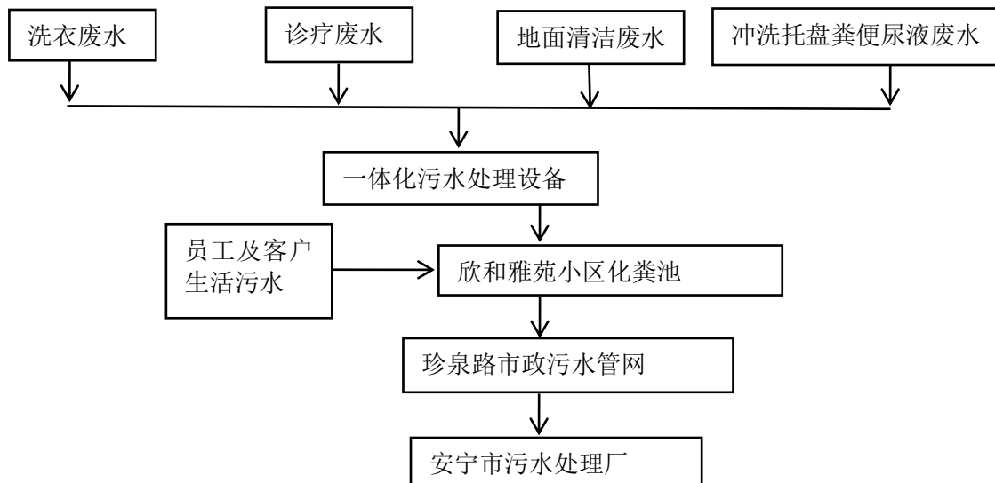
图 4-2 医院污水收集、处理流程
