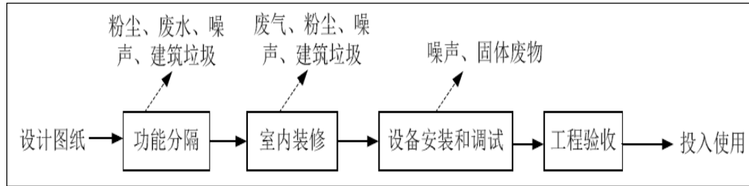
工期工艺流程及产污节点图
