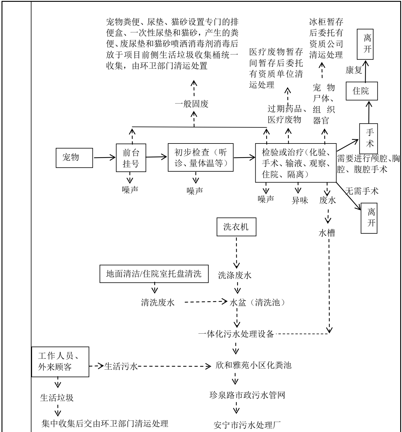
图 2-1 运营期工艺流程及产污节点图
