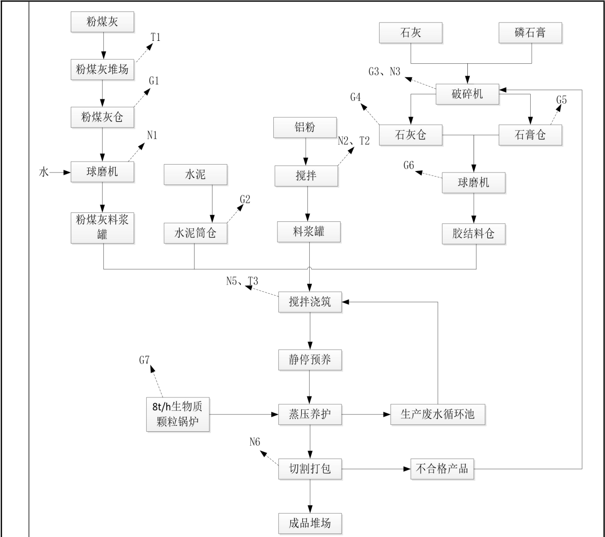
图 2-4 运营期工艺流程图
