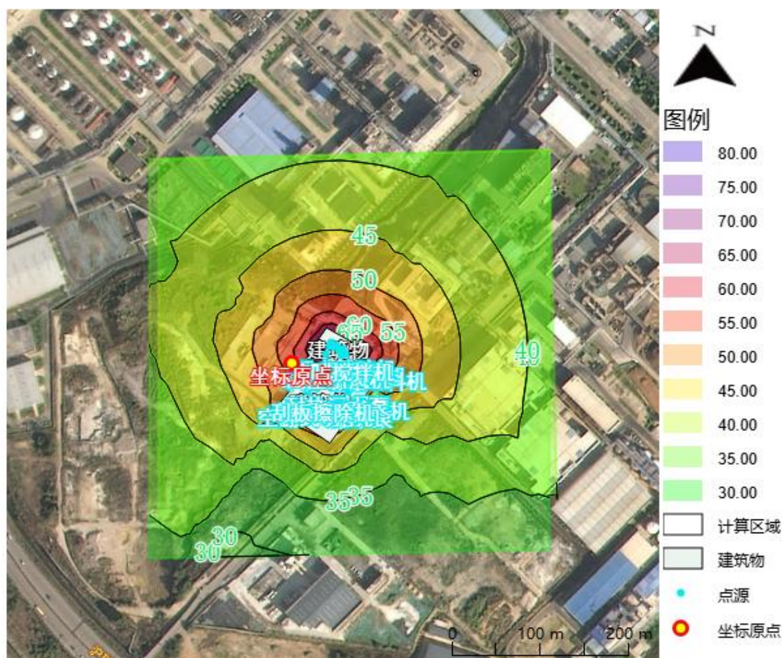
图 4-3 等声级线图
