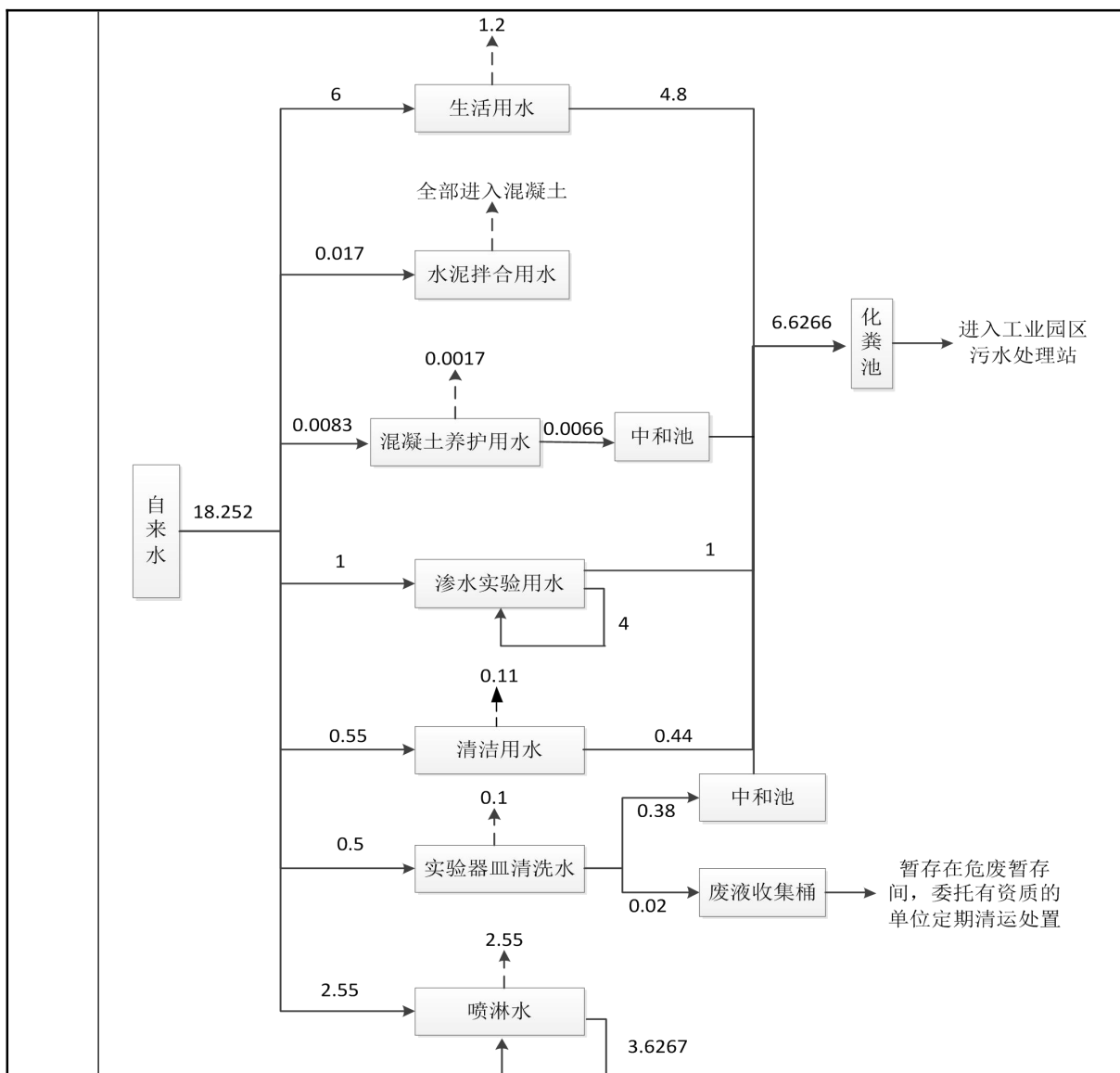
图 2-1 运营期水量平衡图 单位 m³/d
