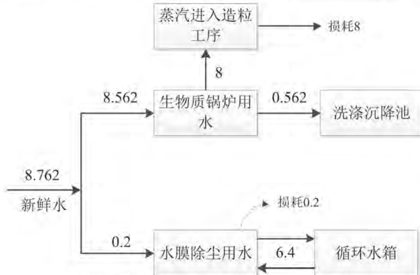
图 4-1 项目运营期锅炉水量平衡图 单位： \text{m}^3/\text{d}
