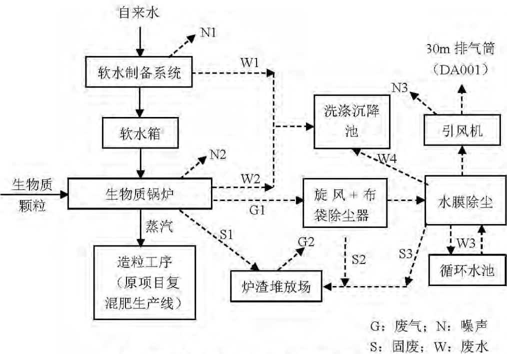
图 2-4 运营期锅炉工艺流程及产污节点图
