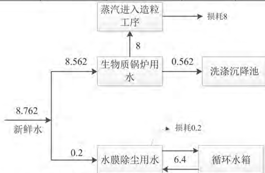
图 2-2 项目运营期锅炉水量平衡图 单位: \text{m}^3/\text{d}
